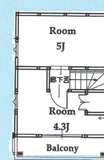
3階 [18.66㎡]
